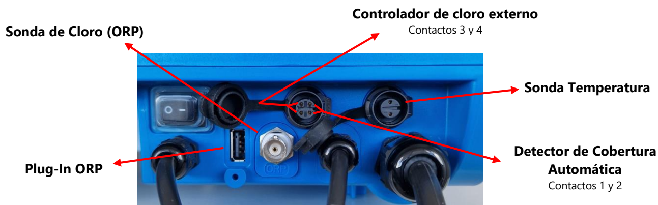
Figura 6 – Conexiones internas
